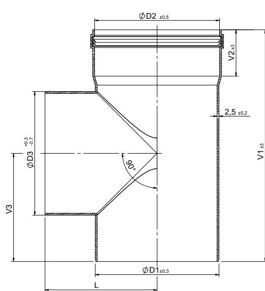
SEC. A-A
