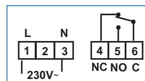
Siesta-TA RF
